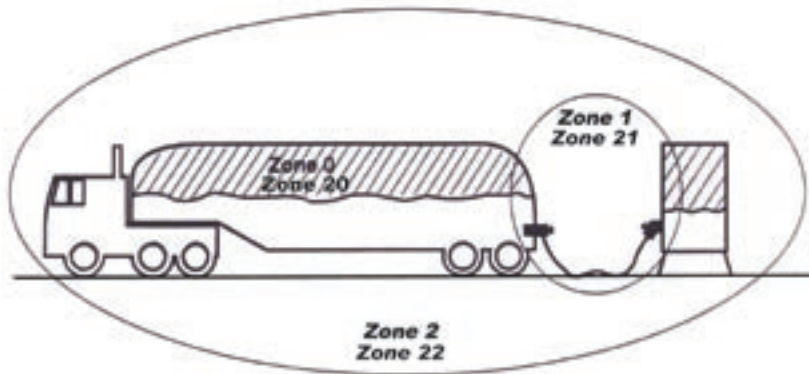
Beispiel für die Zoneneinteilung. Gas: Zone 0, 1 und 2. Staub: Zone 20, 21 und 22.
