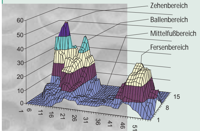
Maximaldruckdarstellung eines Abrollvorgangs auf WERKSTEP-Matten
